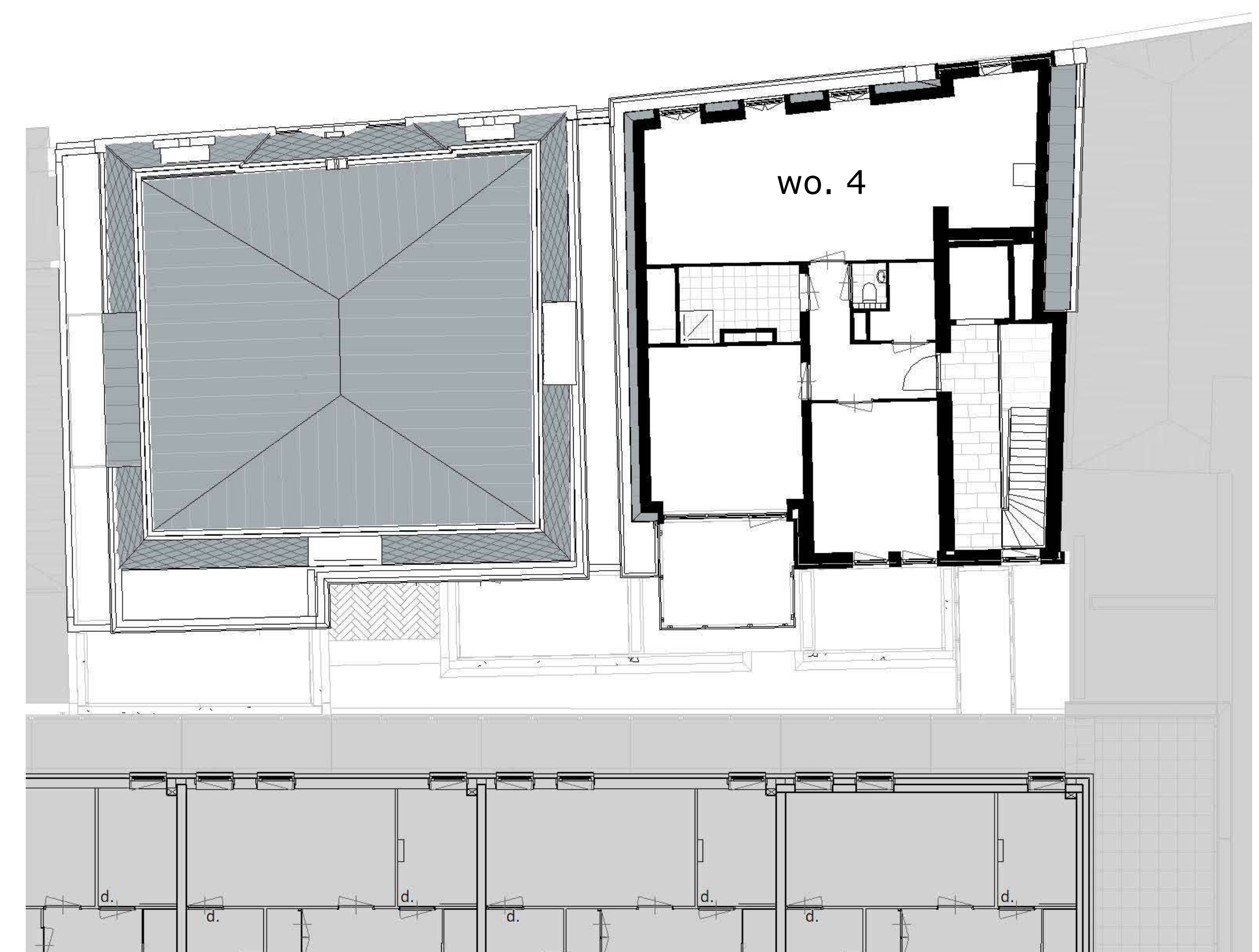
Verdiepingsoverzicht niveau 3
