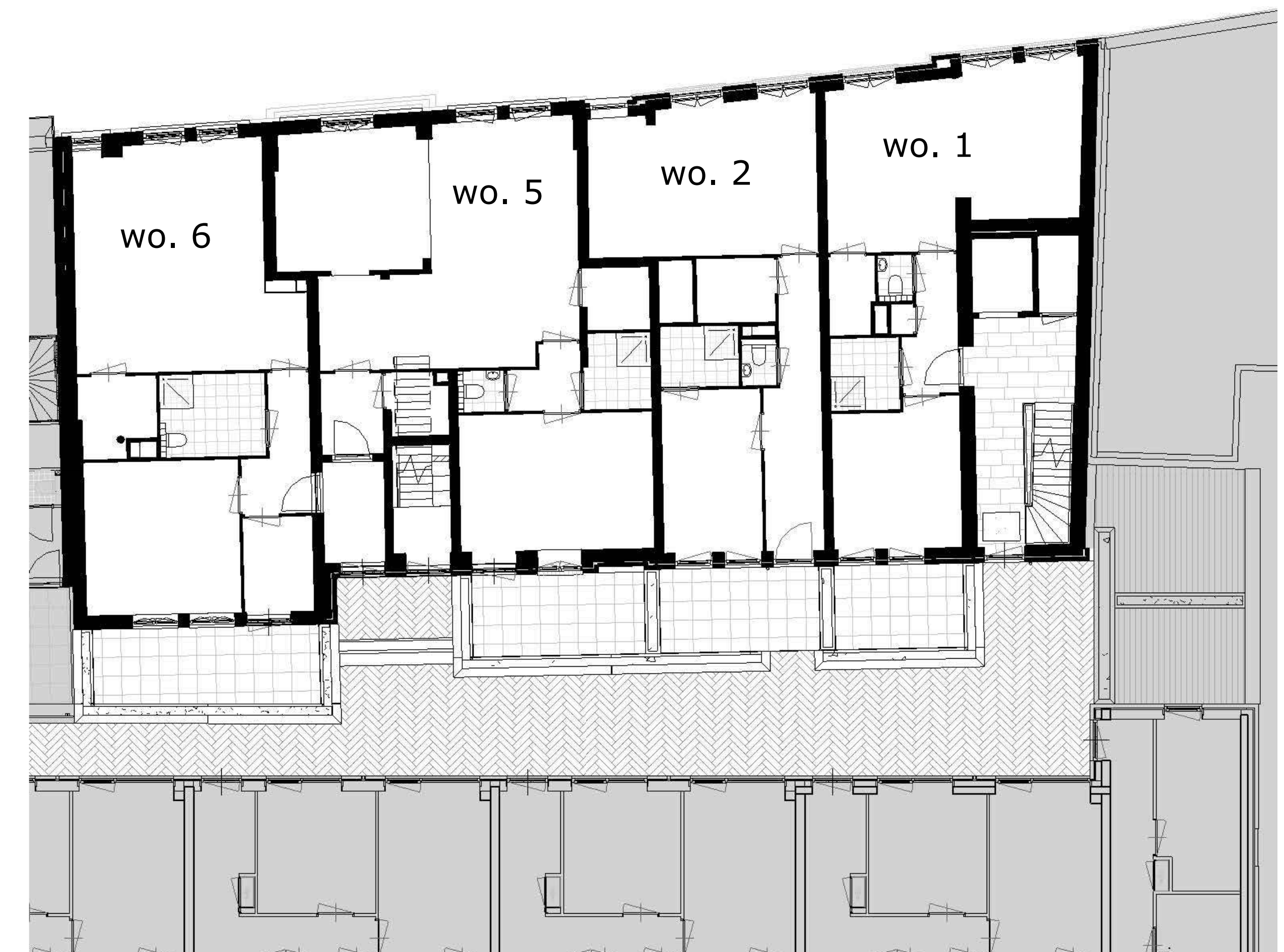
Verdiepingsoverzicht niveau 1
