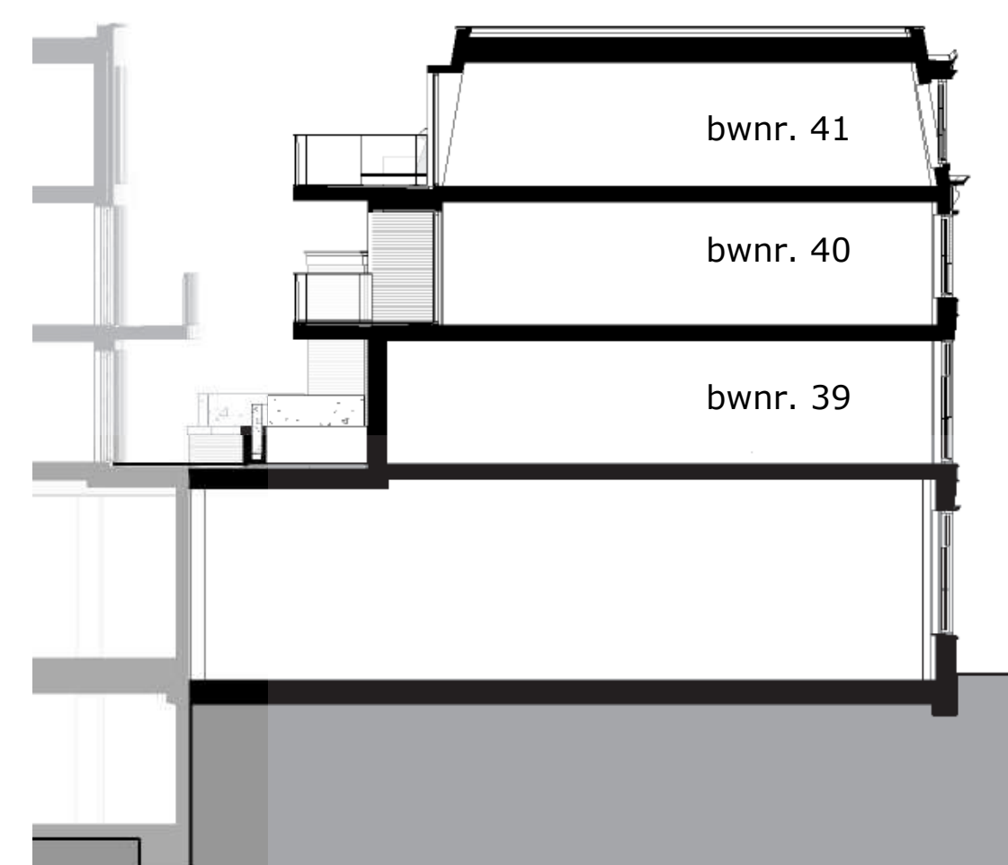
Doorsneden
